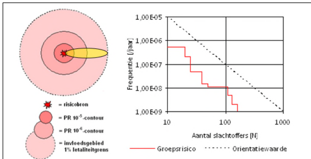
Figuur 2: Weergave plaatsgebonden risicocontouren, invloedsgebied en groepsrisicografiek met oriëntatiewaarde voor een inrichting. Hierbij stelt de gele pluim een toxische wolk voor een bepaalde windrichting.
