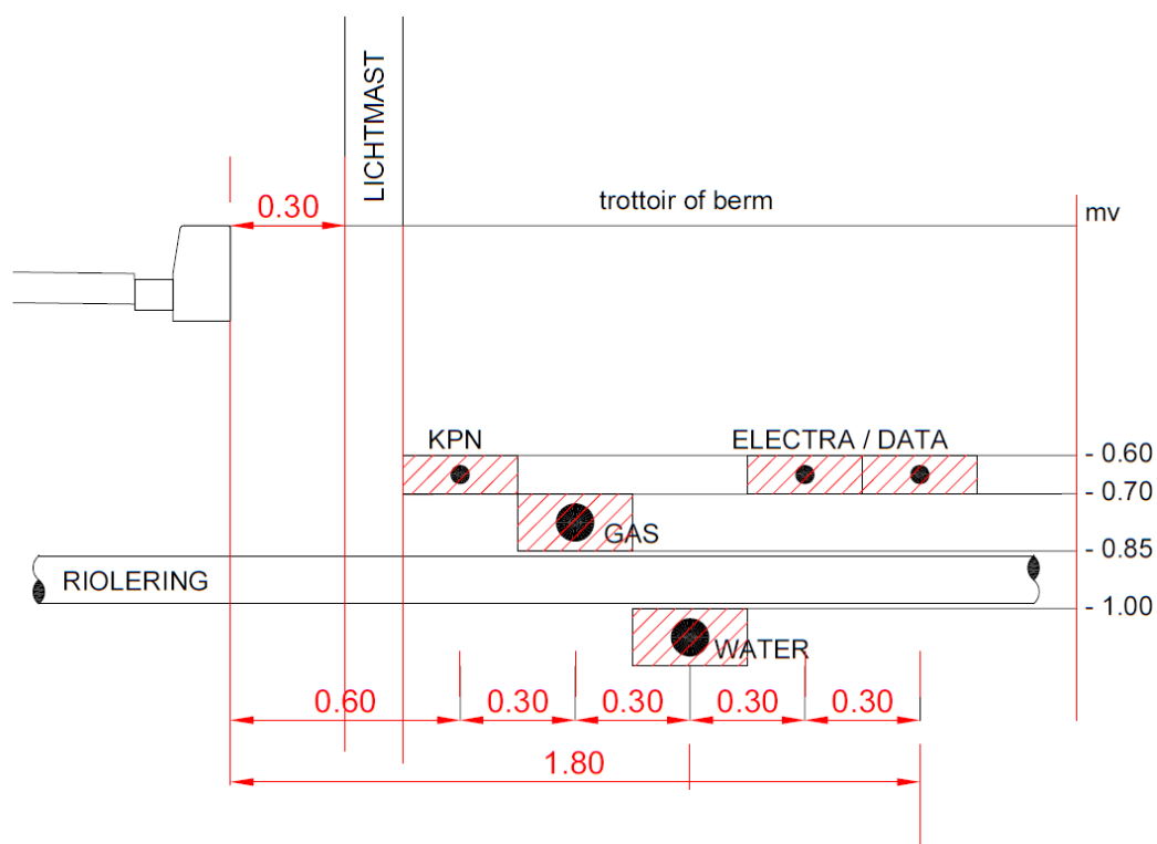
Dwarsprofiel kabel- en leidingschema
